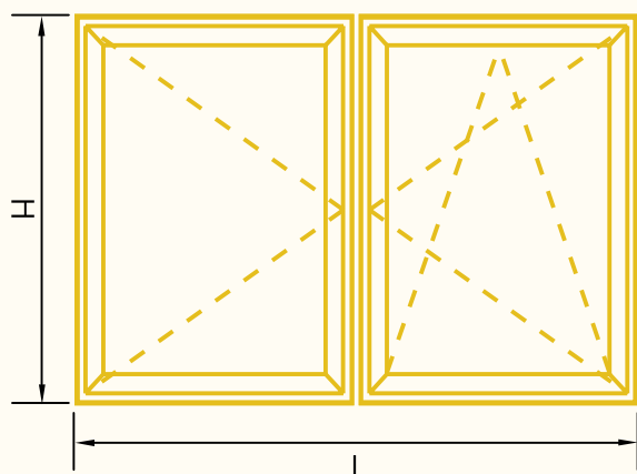
Janela de Abrir de 2 Folhas Abertura Interior
